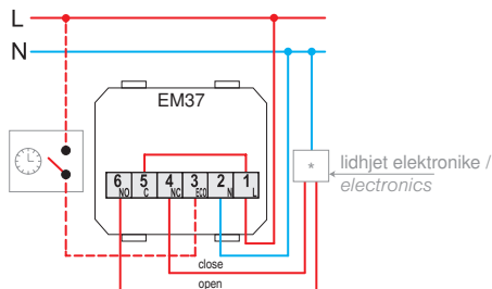
transmisioni me motor (përdorim i kufizuar me ngrohje nën dysheme) / motor drive (limited use with underfloor heating)
