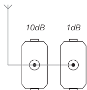
Durchgangsschaltung throughpass connection
